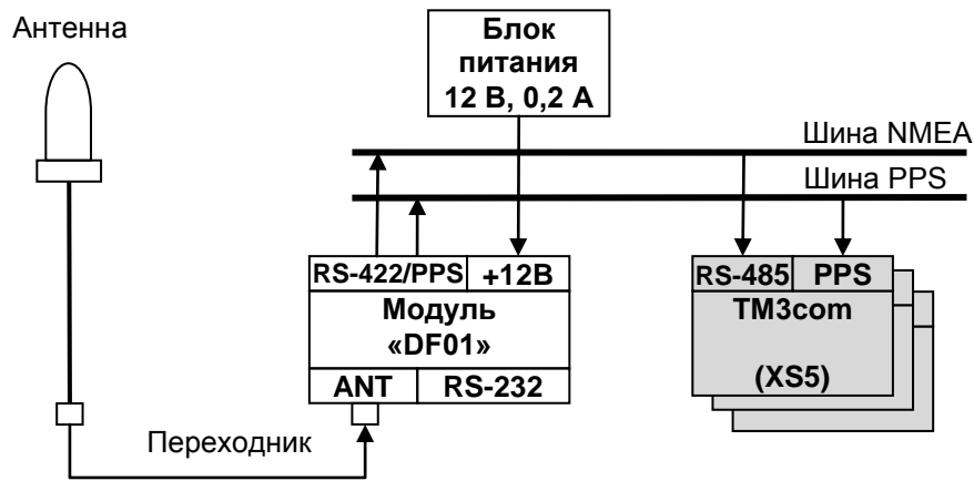
Рисунок 7 – Подключение модуля «DF01» к устройству «ТМ3com»
