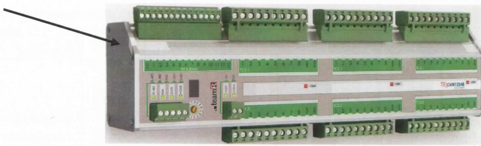
Рис.2 Внешний вид блока ввода ТС/ТИТ ТЕ306N12S48 и место опломбирования после поверки.
